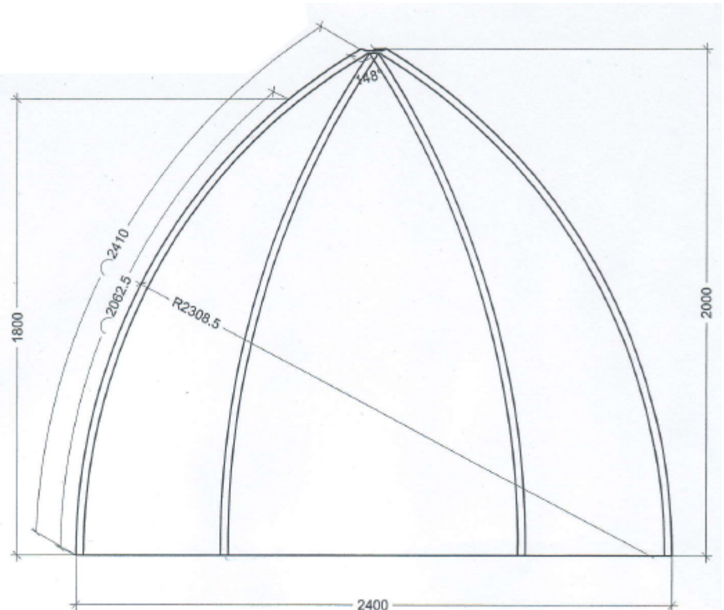
Ansicht (M 1:25)
